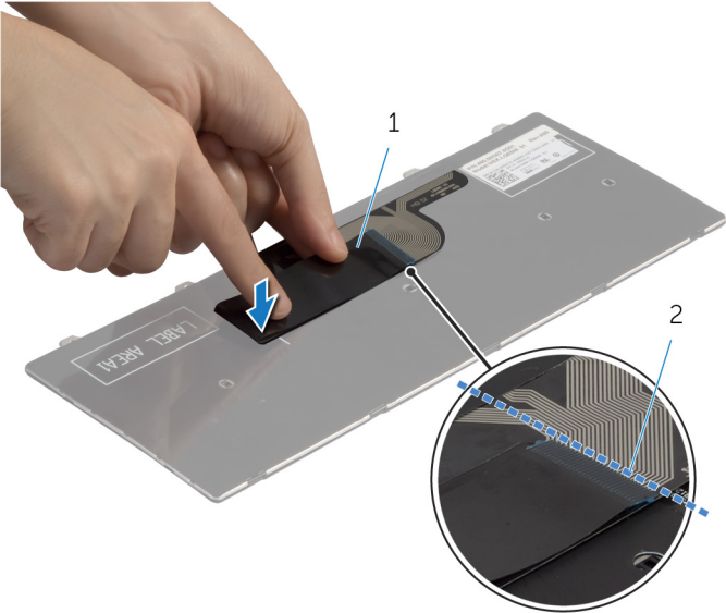
1 键盘电缆
