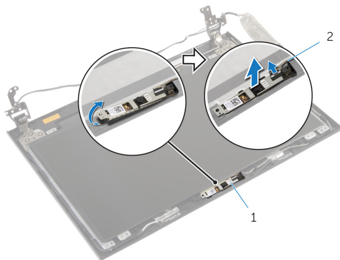
1 摄像头
