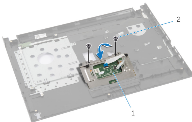
1 触摸板
